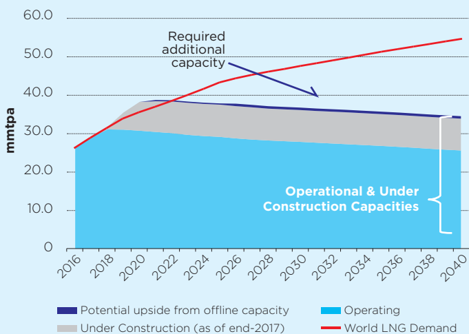
Effective Liquefaction Capacity vs. LNG Demand
